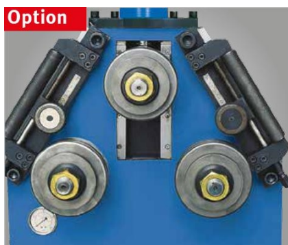
Opcjonalnie specjalne rolki prowadzące na bokach do kątowników
