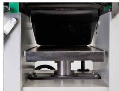
Regulacja stołu grubościówki poprzez pokrętkę ręczną, skalę i wyświetlacz numeryczny.
